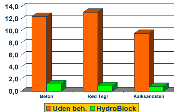
Grafen viser den effekt HydroBlock har på reduktion i vandoptagelsen på forskellige materialer. Før og efter behandling med HydroBlock.
